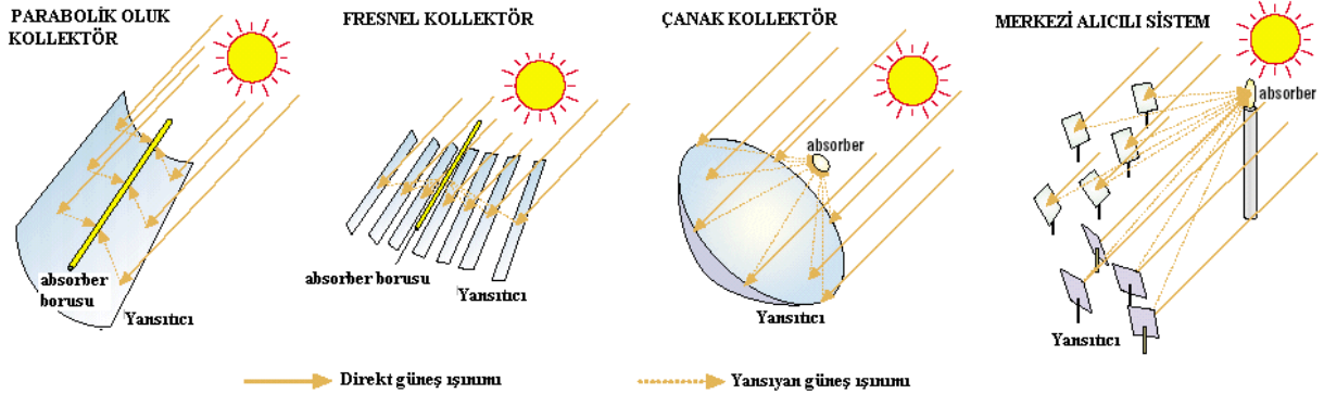
Şekil 20. Yoğunlaştıran güneş enerjisi teknolojileri şematik çalışma prensibi
