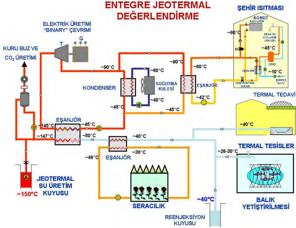
Şekil 11. Jeotermal enerjinin entegre kullanımı.
