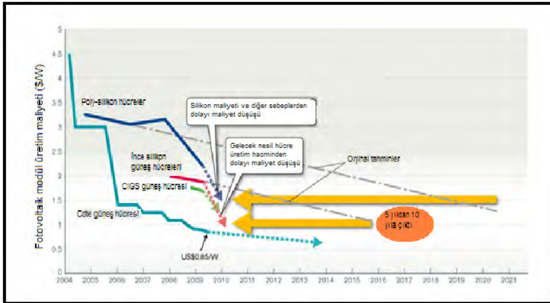
Şekil 9. (a) Polisilikon malzeme fiyatındaki ani düşüşün modül üretim maliyetlerine yansımaları 9 , (b) Modül üretimlerinde tahminlerden önce beklenen maliyet düşüşleri 9 .
